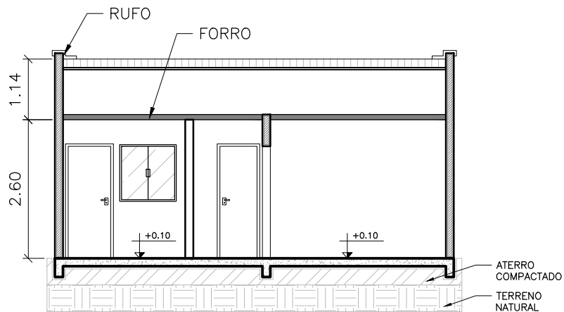
04 CORTE BB - TRANSVERSAL ESCALA 1:100
